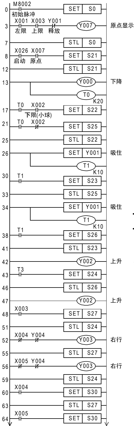
《步进梯形图》
