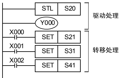
《步进梯形图》
