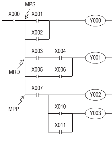
梯形图程序
