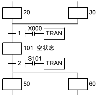
《SFC程序》
