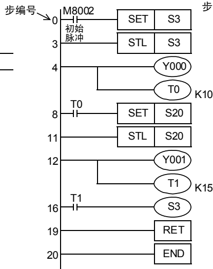
《步进梯形图》
