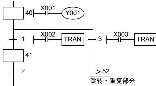
《SFC程序》
