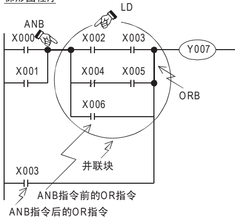
梯形图程序
