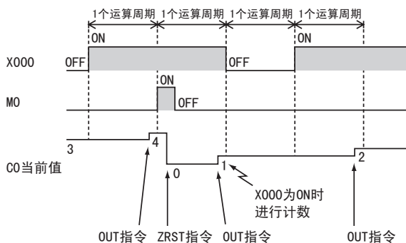
时序图
