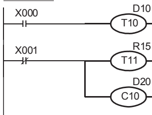
梯形图程序
