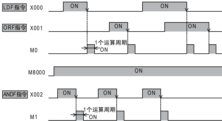
时序图
