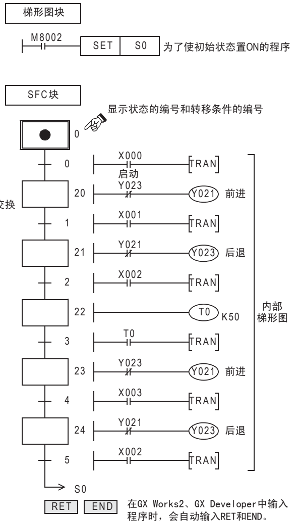
《SFC程序》
