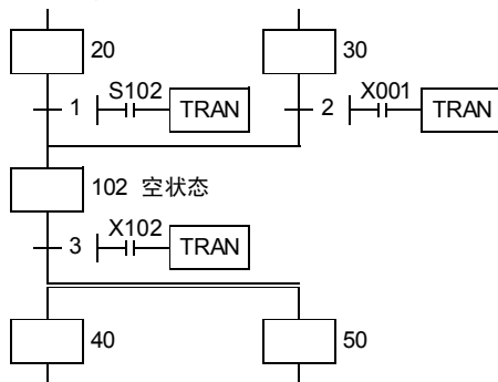
《SFC程序》
