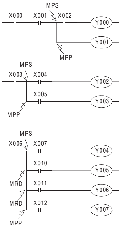
梯形图程序
