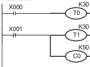
梯形图程序
