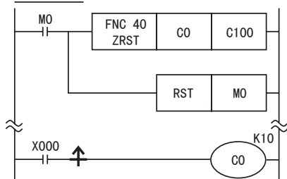
梯形图程序
