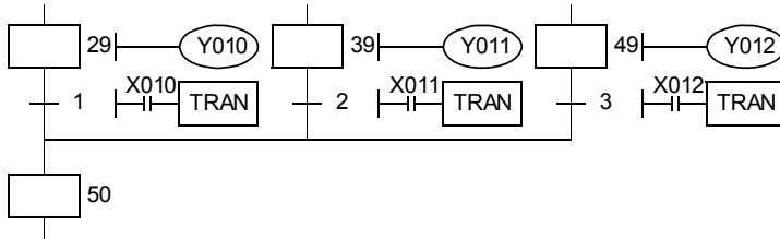
《步进梯形图》
