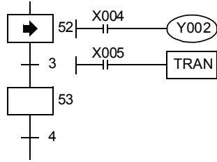
《SFC程序》
