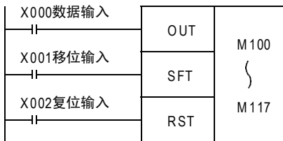
梯形图程序
